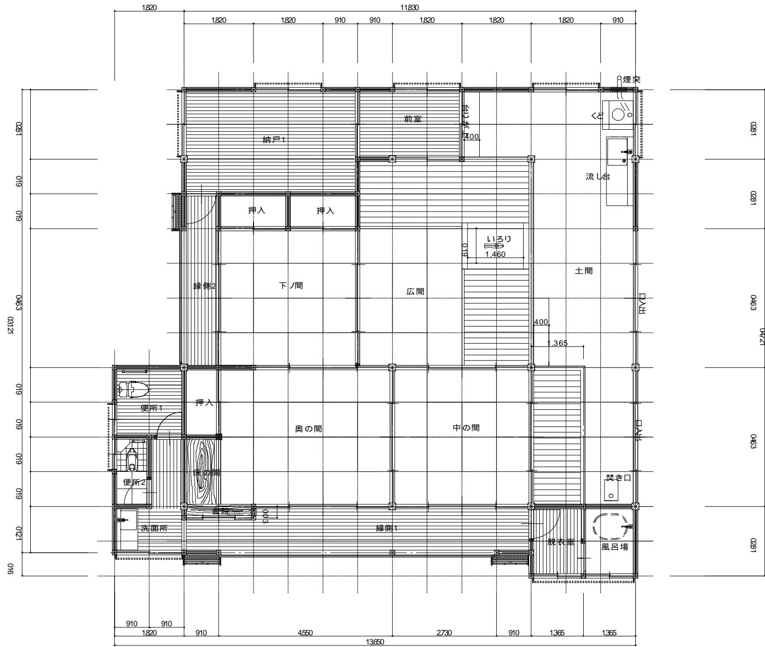
平面図 1/50
